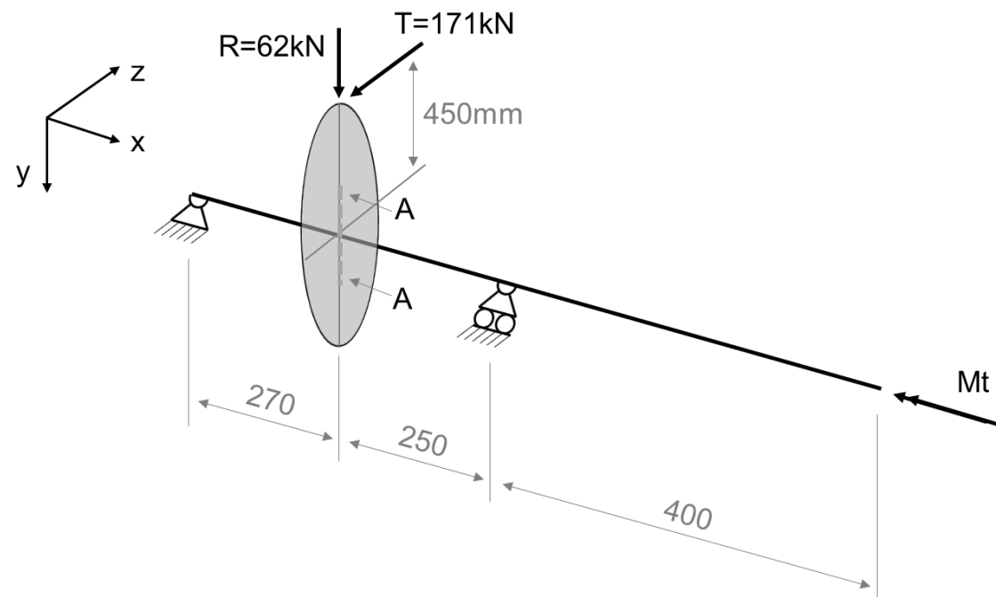
Fig. 2. Schema albero lento riduttore (ruote dentate a denti diritti).
