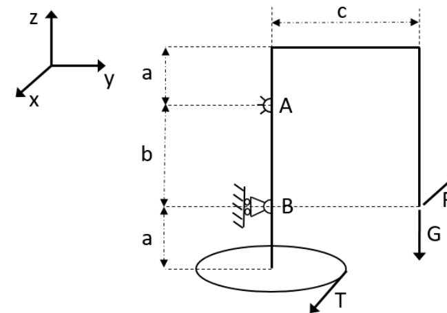
Figura 1: Schematizzazione struttura agitatore.
