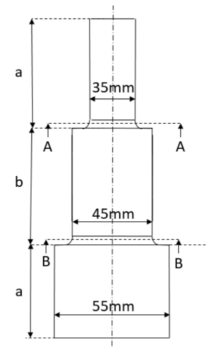
Figura 2: Schematizzazione albero principale.
