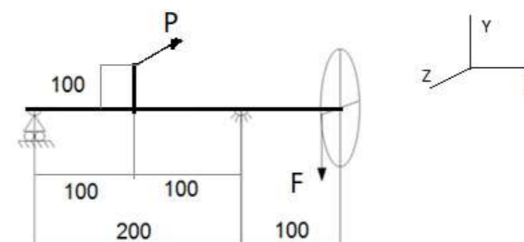
Fig. 1. Schema della trasmissione. Misure in mm.
