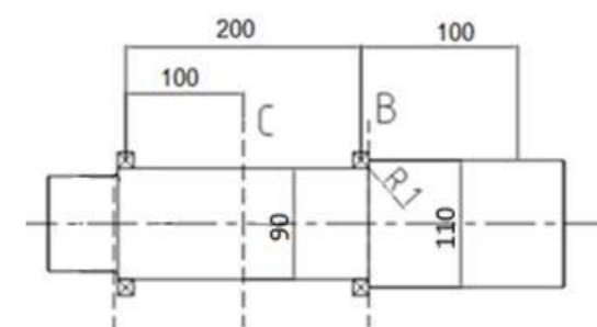
Fig. 2. Schema e quote in mm dell'albero.
